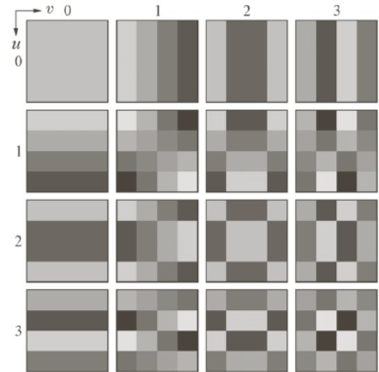
n=4时的DCT的基函数
